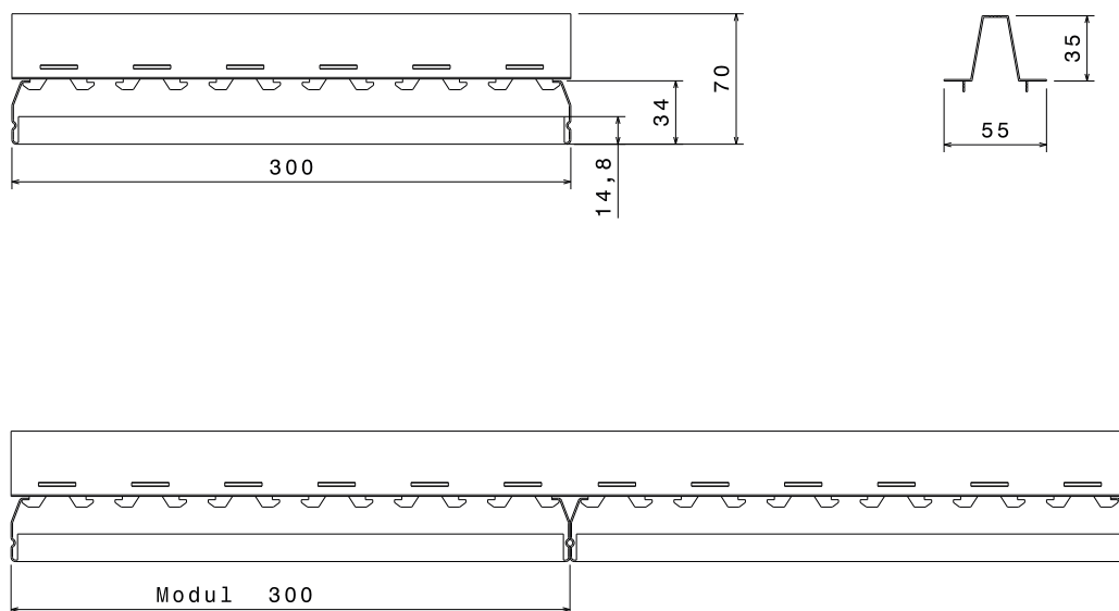
Trageschiene Typ HZF
